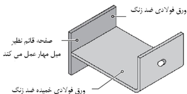
شکل ۴-۱۴- بست‌های ترکیبی بار ثقیل و جانبی شامل ورقه فولادی ضد زنگ
