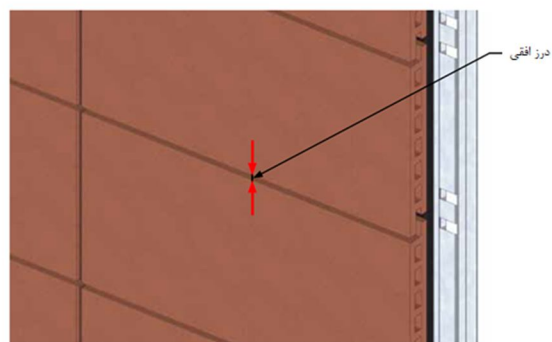
شکل ۷-۱۶- کنترل ایجاد درز عمودی ثابت و صاف
