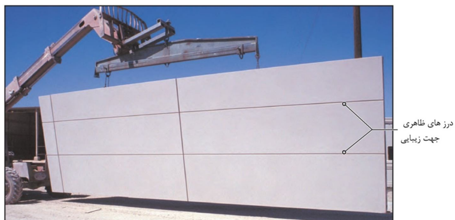
شکل ۶-۳۷ الف - سطح بیرونی یک پانل GFRF، در حال حمل در کارگاه
